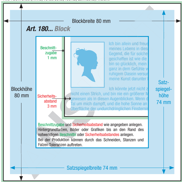
Art. 180... Block, links, Vorderseite, rechts, Leimseite, Ansicht
